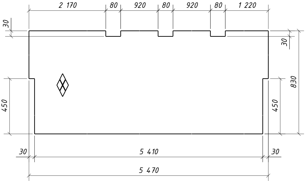
Дет. 1278
