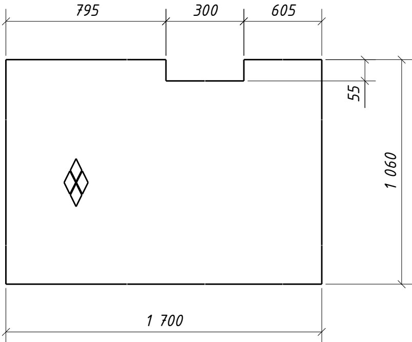
Дет. 1381
