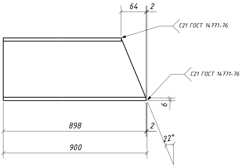
Дет. 1498
