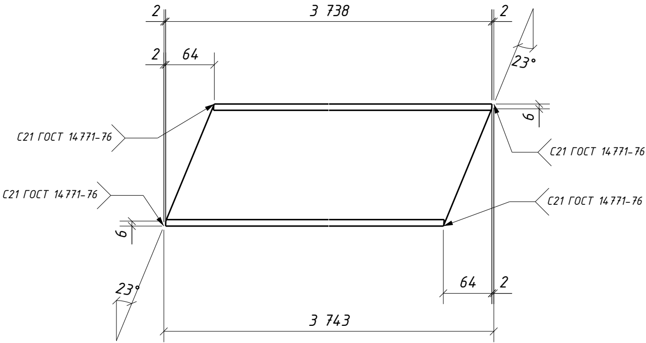
Дет. 1509
