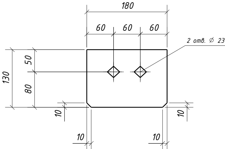
Дет. 1593
