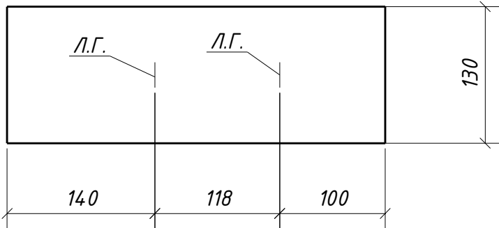
Развертка дет. 1608
