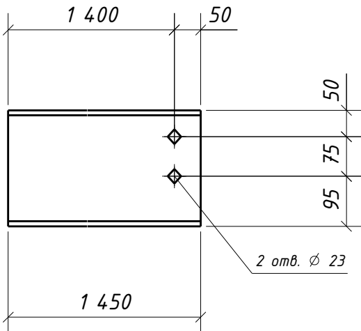
Дет. 1622
