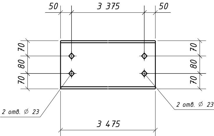
Дет. 1623
