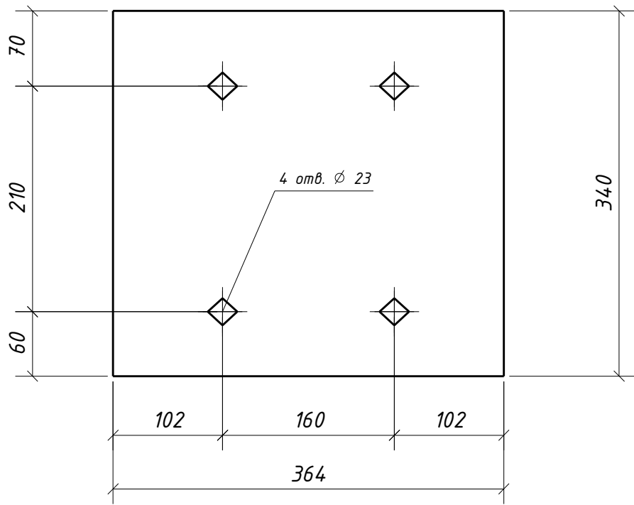
Дет. 1635
