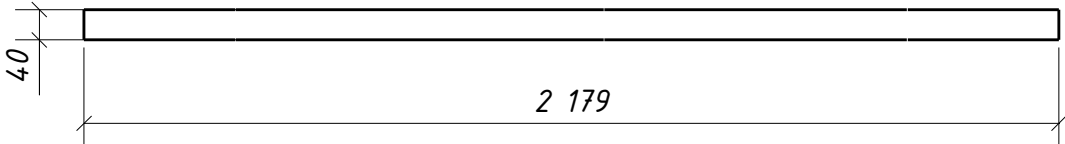
Развертка дет. 1687
