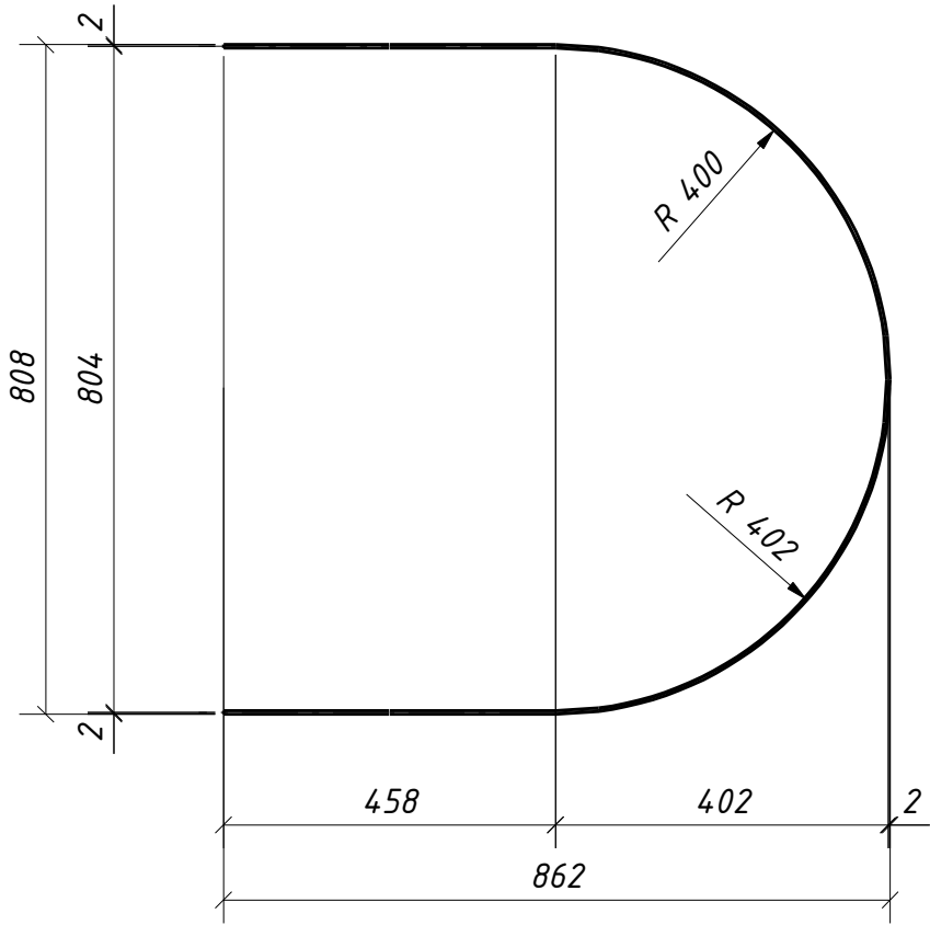
Гиб дет. 1687
