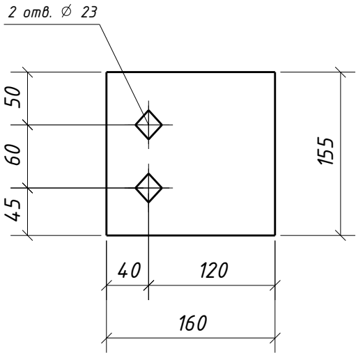
Дет. 233
