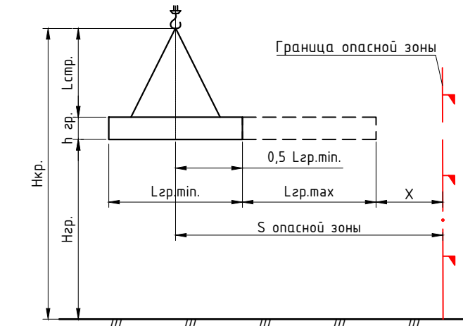
Монтаж профлиста М1:150 Телескопический, коленчатый подъемник +11,450 15,10 -0,150 Ур.з. Автомобильный кран КС-55729-5В (вспомогательный)
