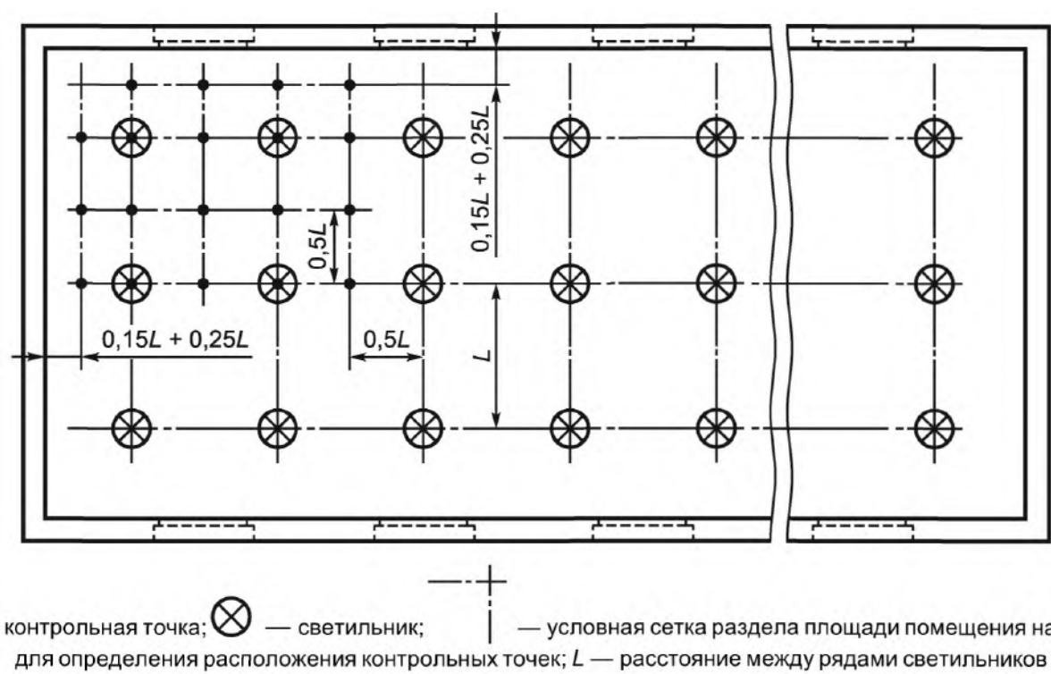
Рисунок 6.17.2. Расположение контрольных точек при измерении минимальной освещенности помещения от светильников, принимаемых за точечные излучатели
