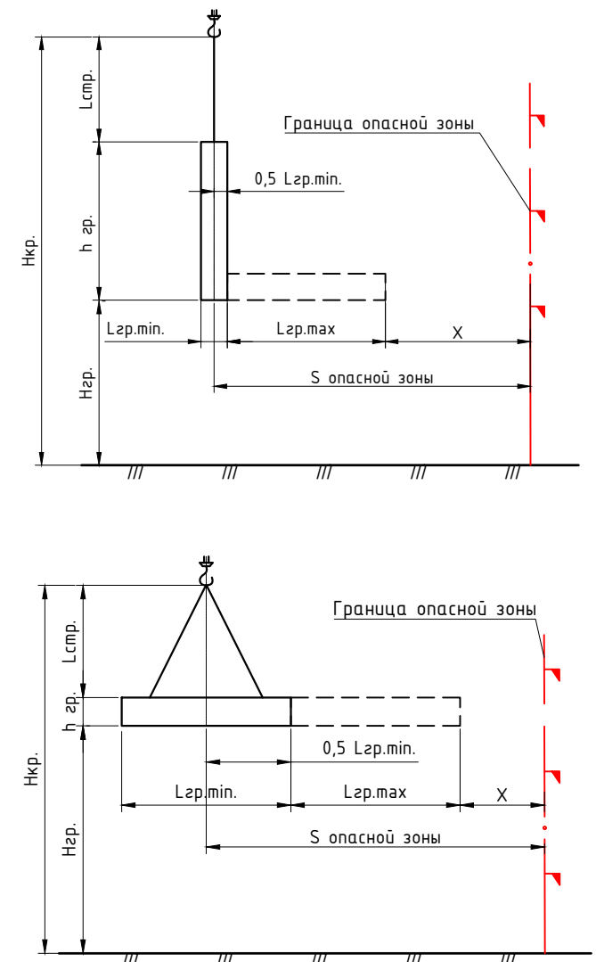
Сигнальное ограждение по контуру опасной зоны
