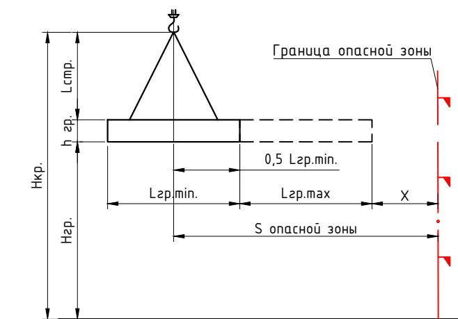
Монтаж профлиста М1:150 Телескопический, коленчатый подъемник Автомобильный кран КС-55729-5В (вспомогательный) +11,450 15,10 -0,150 Ур.з.
