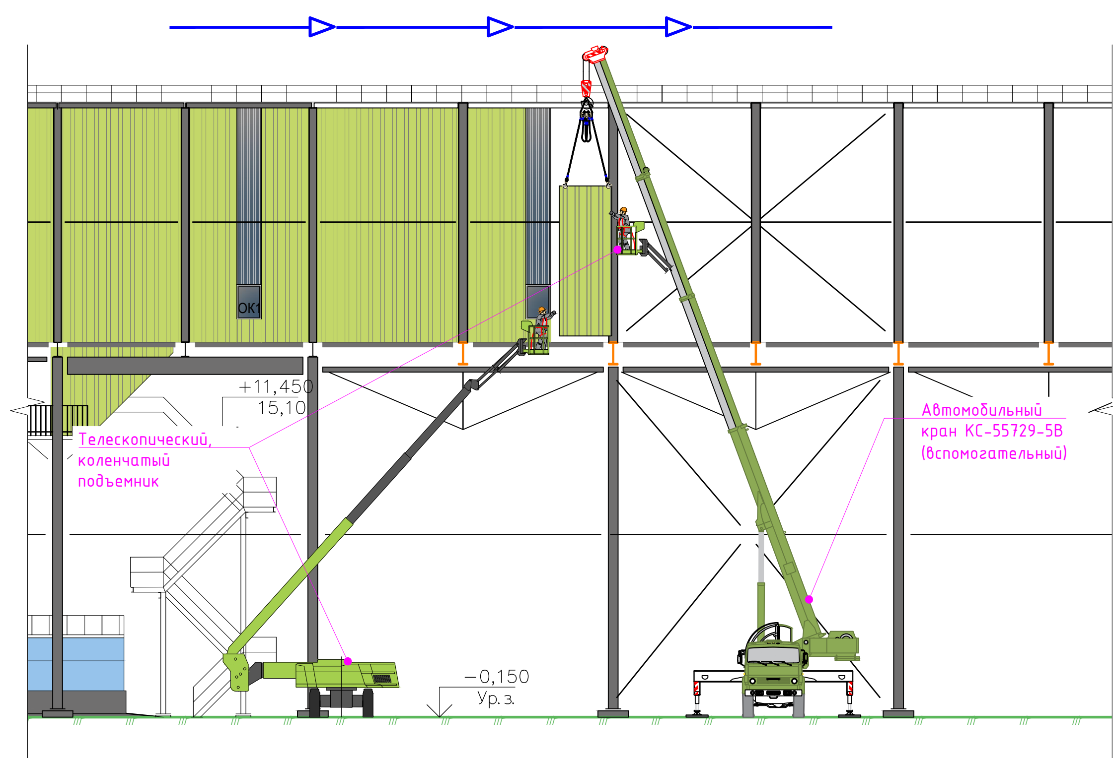
Монтаж профлиста М1:150
