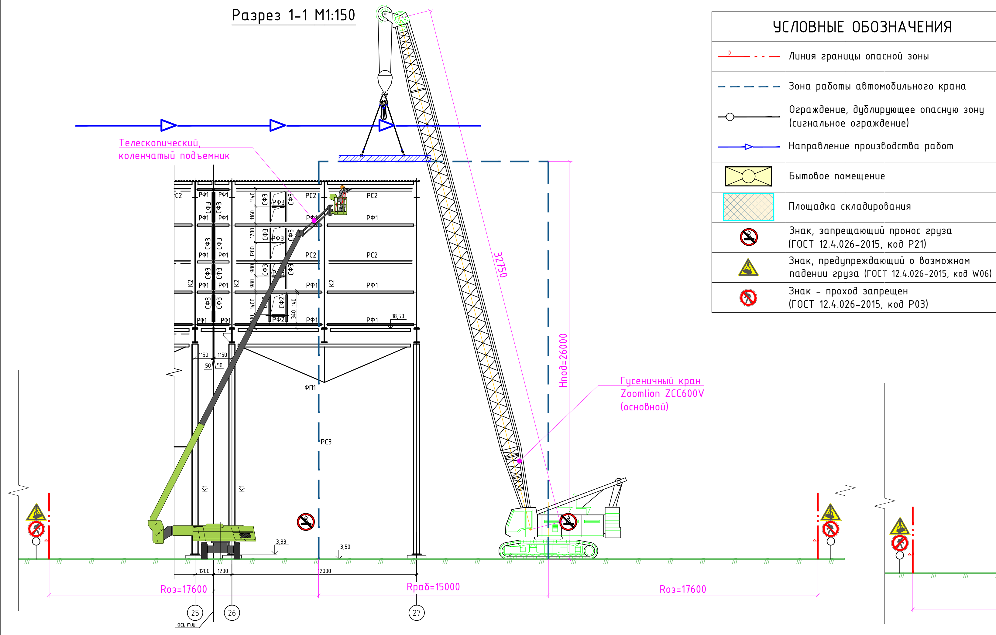
Разрез 1-1 М1:150
