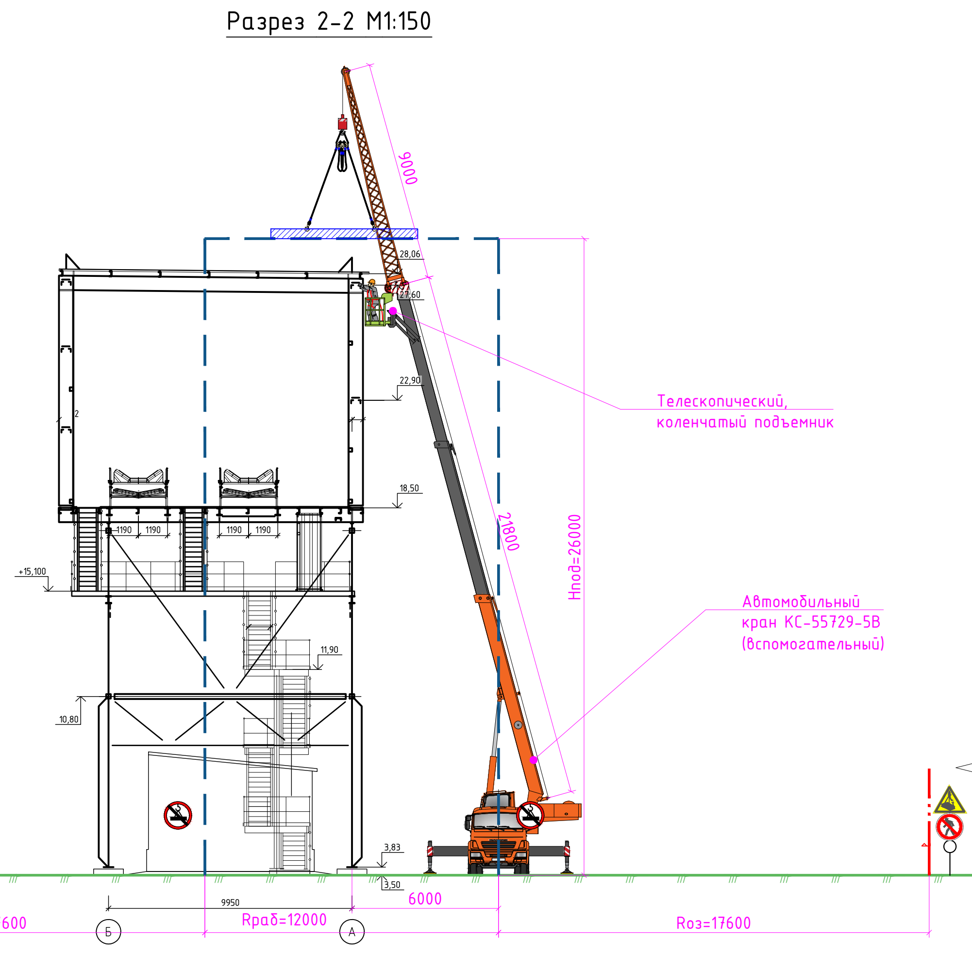
Разрез 2-2 М1:150
