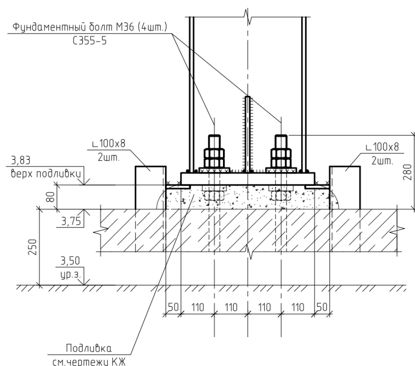
Рисунок 15.2.7. Принципиальная схема монтажа колонн
