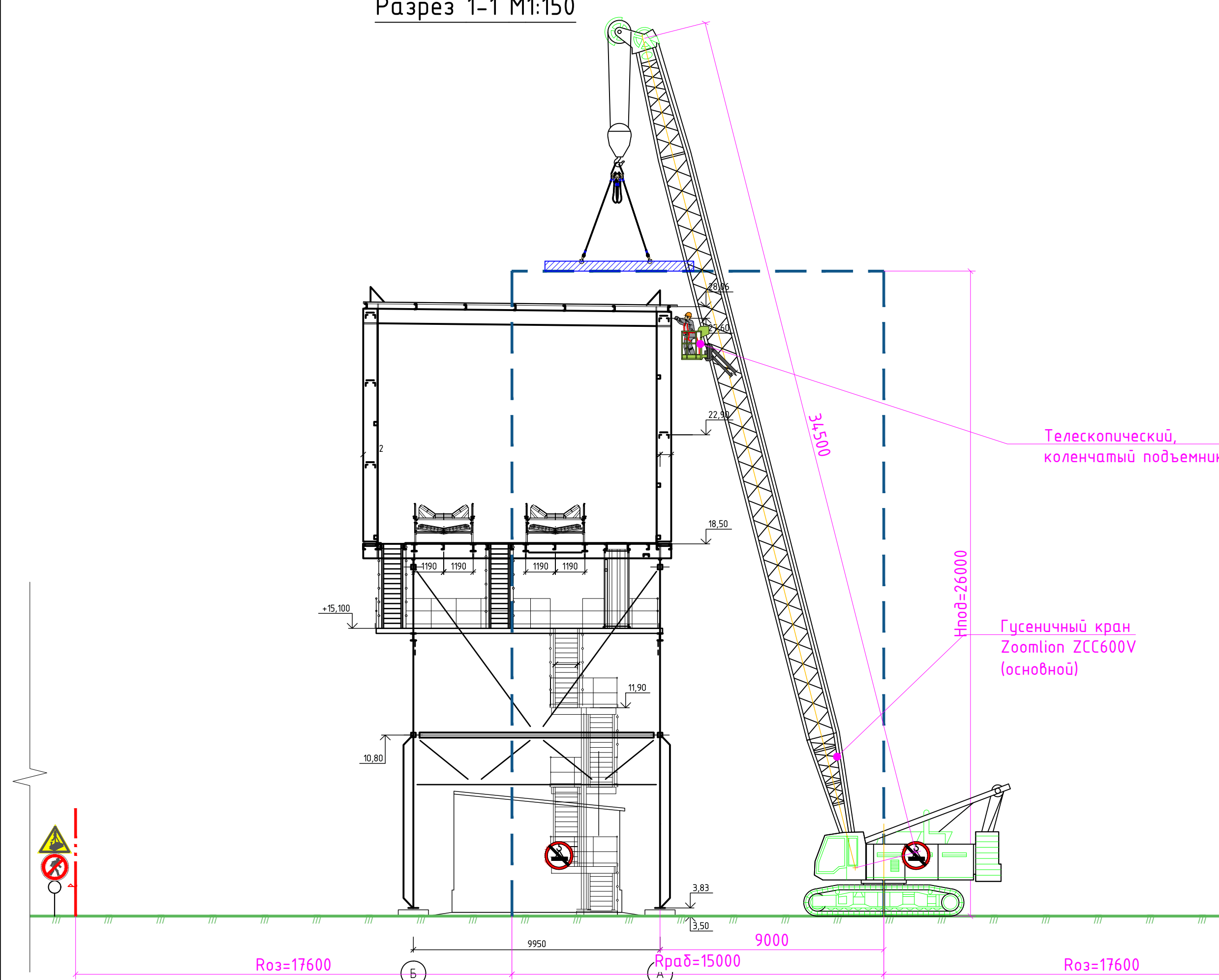
Разрез 1-1 М1:150
