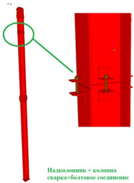
Рисунок 15.2.3. Укрупнительная сборка колонн и надколонников
