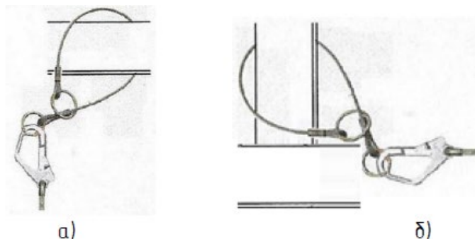
Рисунок 15.2.11. Крепление анкерного стропа: за горизонтальную металлоконструкцию (а), за вертикальную металлоконструкцию (б).
