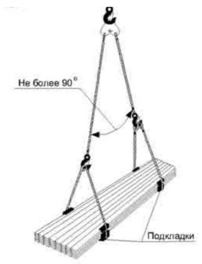
Рисунок 15.2.9. Строповка пачки профилированного листа при разгрузке
