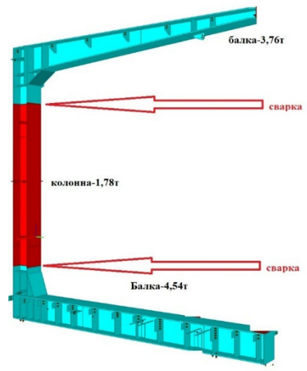
Рисунок 15.2.6. Укрупнительная сборка С-образного элемента
