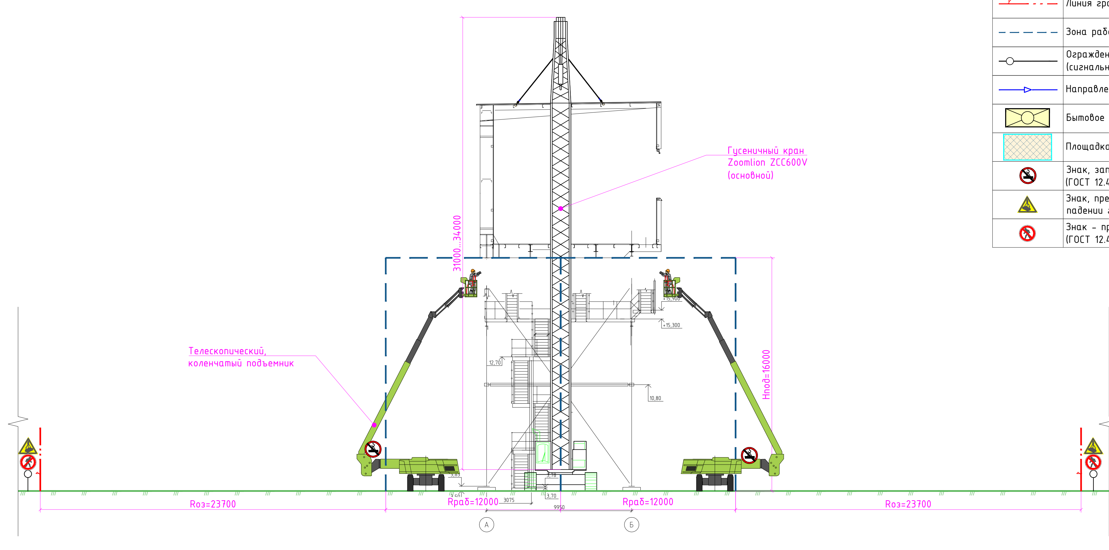
Разрез 2-2 М1:50
