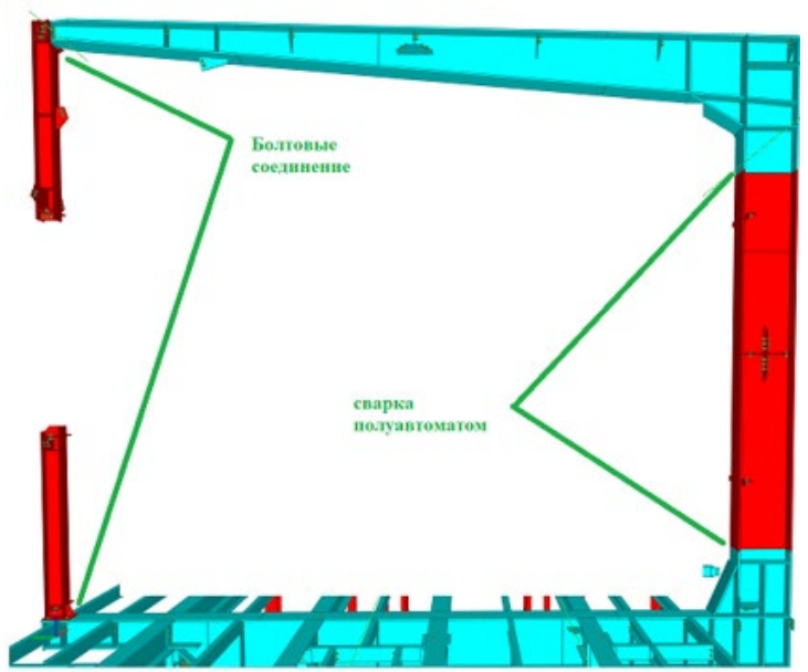
Рисунок 15.2.4. Укрупнительная сборка С-образного элемента
