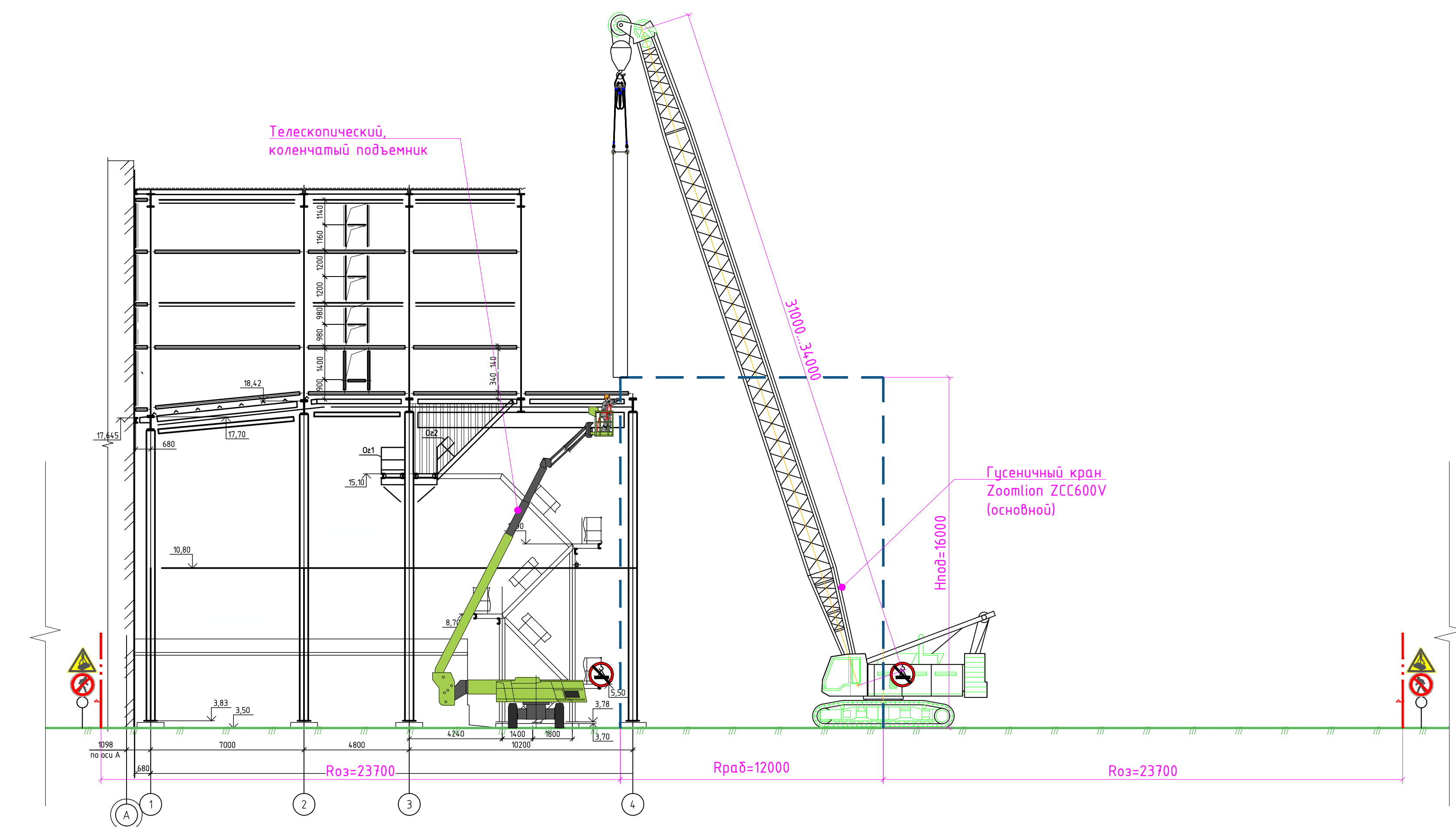
Разрез 1-1 М1:50
