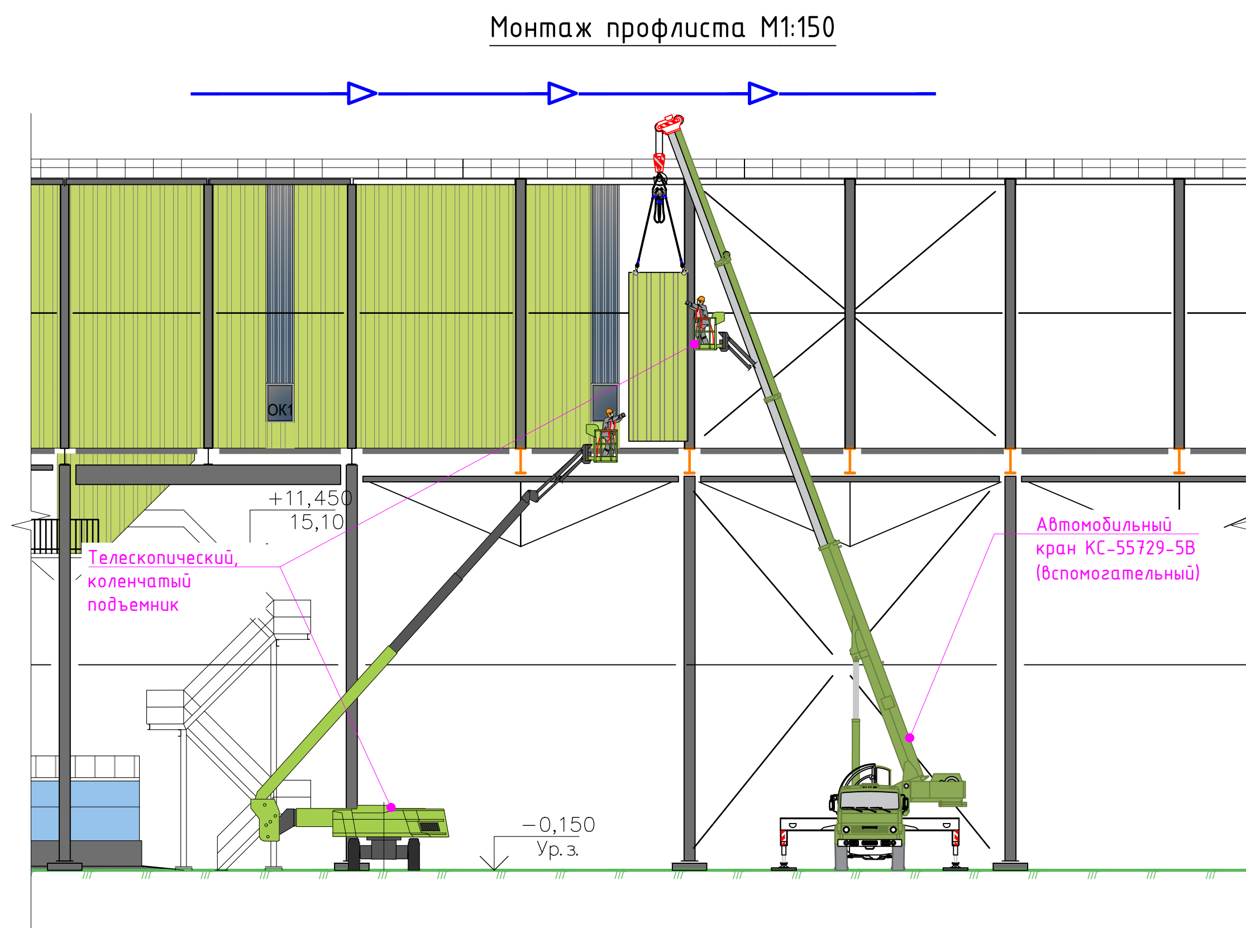
Монтаж профлиста М1:150
