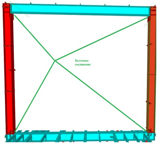
Рисунок 15.2.5. Укрупнительная сборка О-образного элемента
