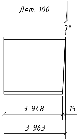
Вид снизу
