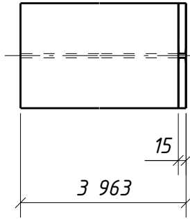
Вид снизу
