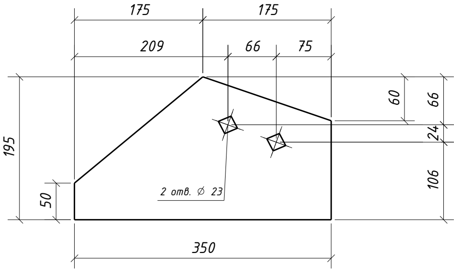
Дет. 118
