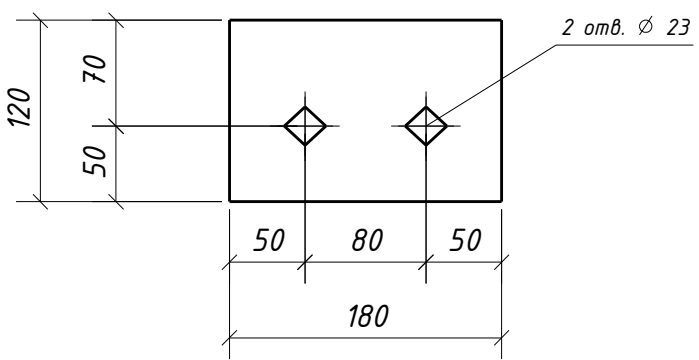
Дет. 132
