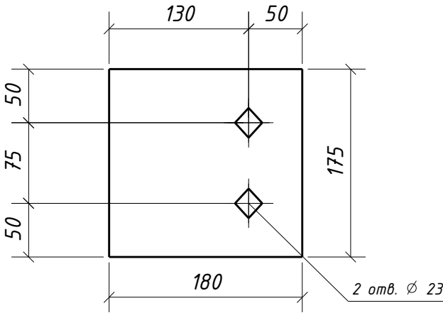
Дет. 134
