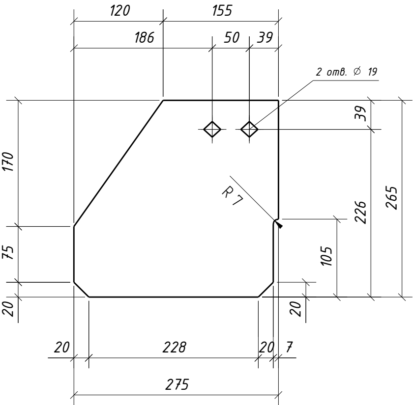
Дет. 177
