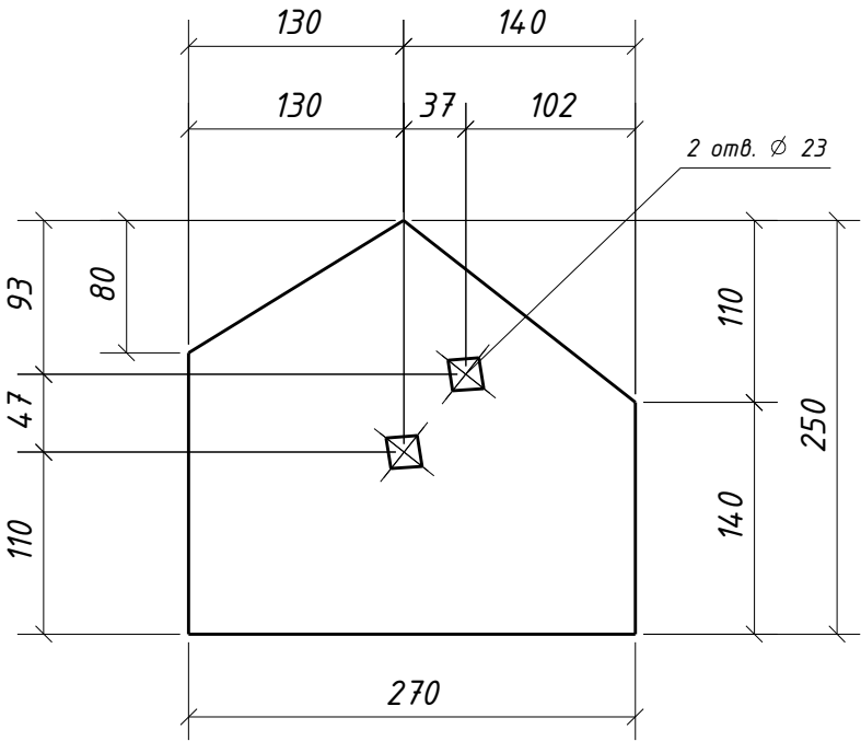
Дет. 190
