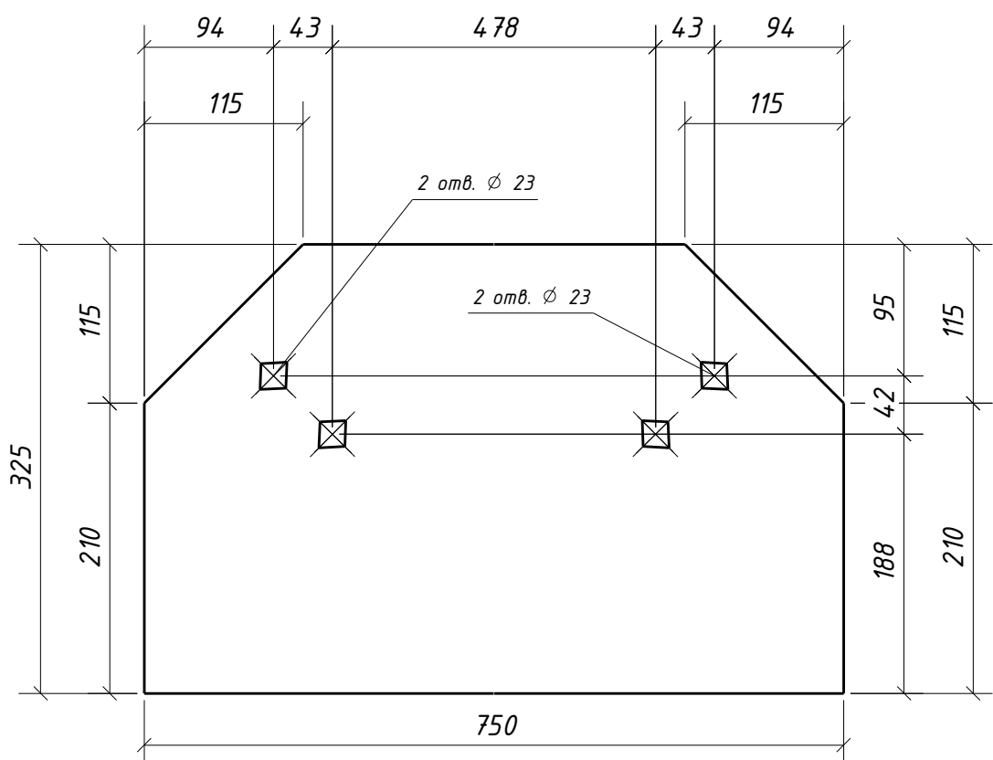
Дет. 249
