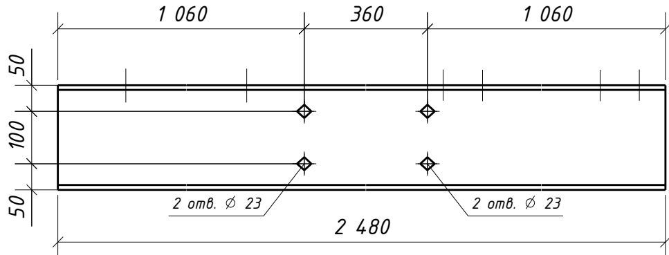
Дет. 275
