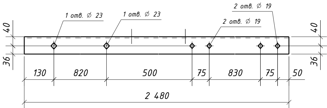
Дет. 275
