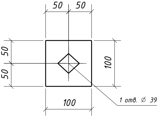
Дет. 311
