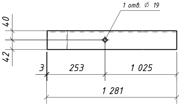
Вид сверху
