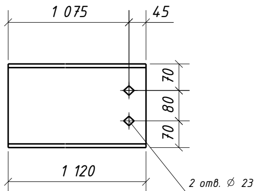
Дет. 371
