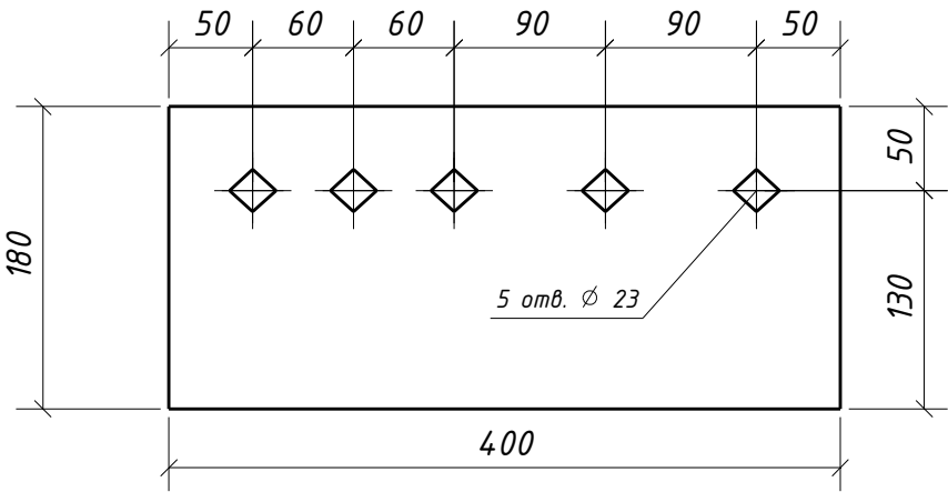
Дет. 49
