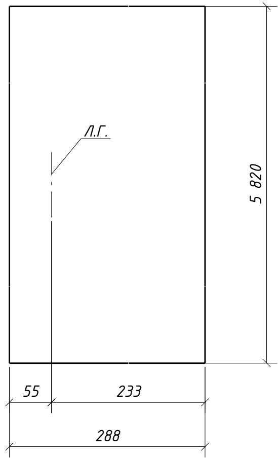
Развертка дет. 627
