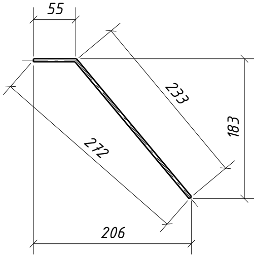
Гиб дет. 627
