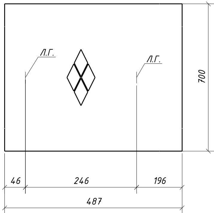
Развертка дет. 672
