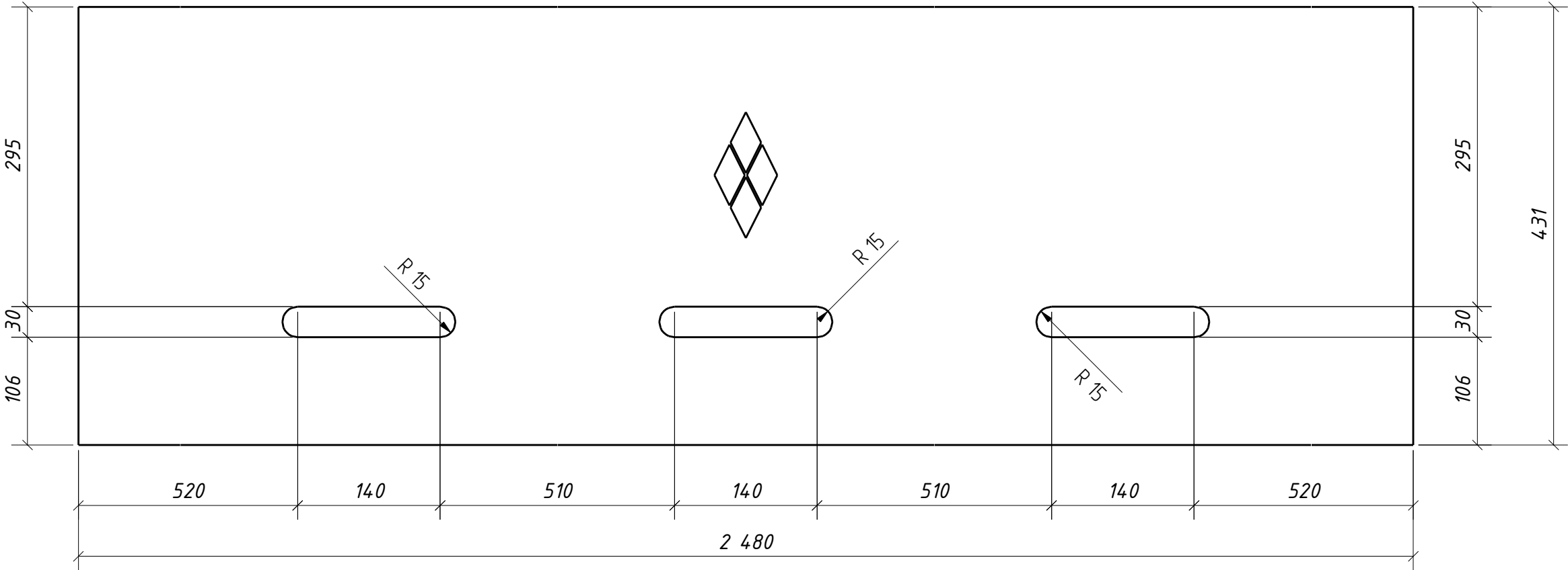
Дет. 677
