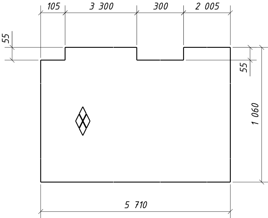
Дет. 824
