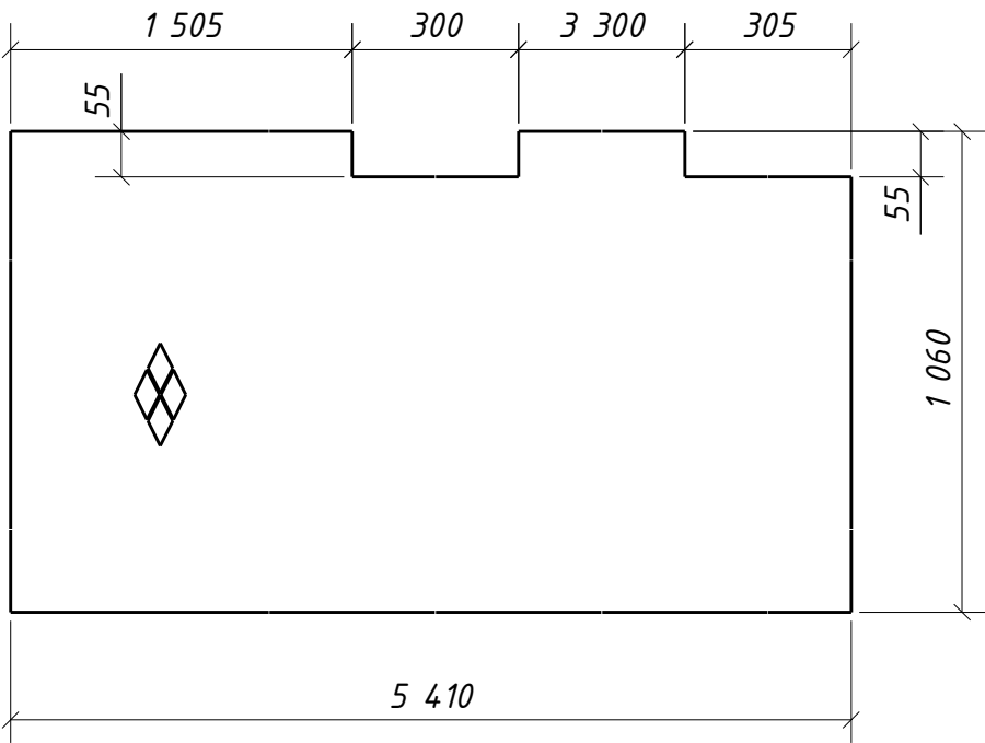
Дет. 829
