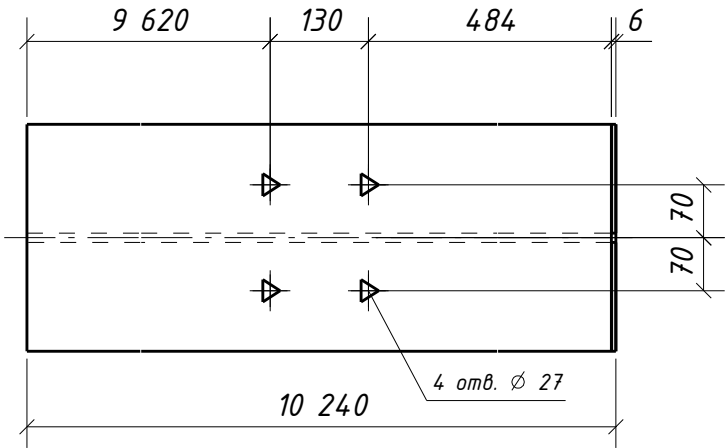
Вид сверху
