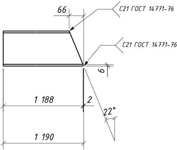
Дет. 879
