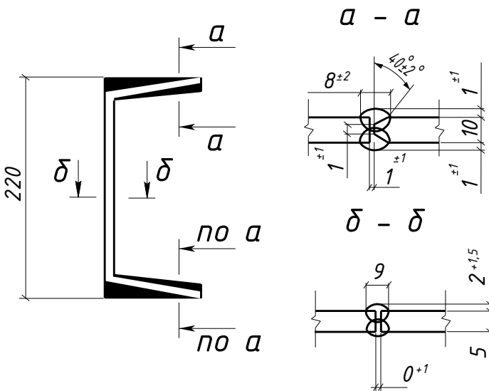
Типовой стык для Швеллер22П/У швы с полным проваром УЗК-100%
