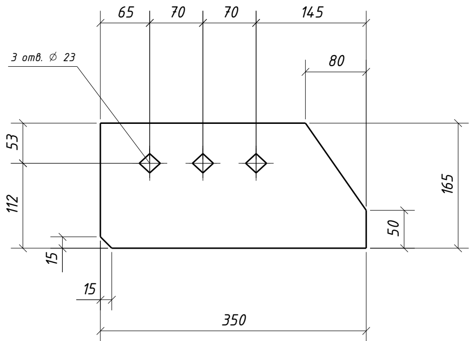
Дет. 102
