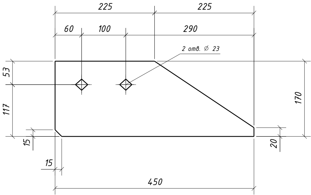
Дет. 1094
