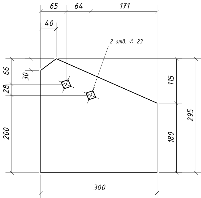
Дет. 1103
