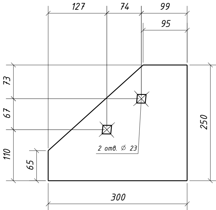
Дет. 1121
