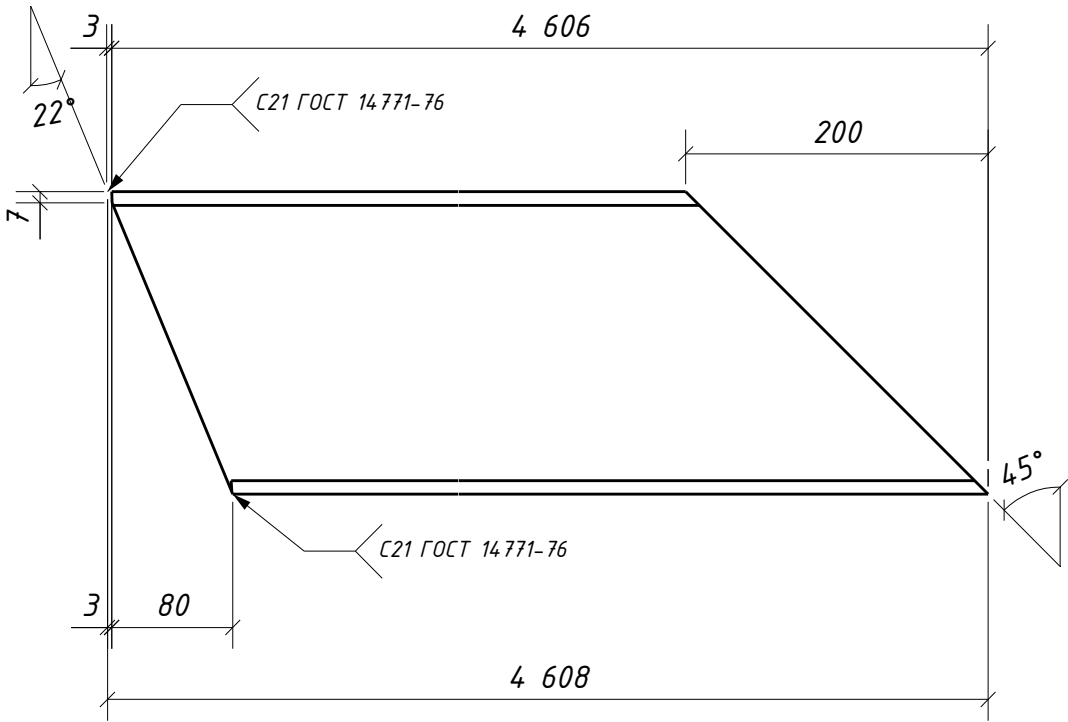
Дет. 1206
