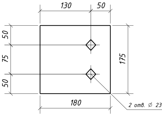
Дет. 134
