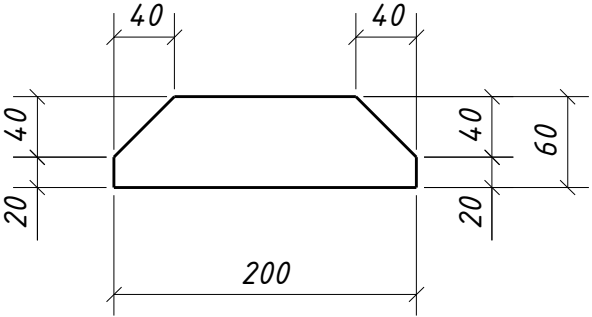
Дет. 203
