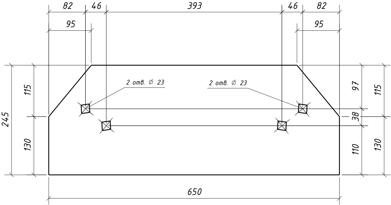
Дет. 245
