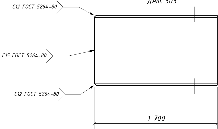
Дет. 303
