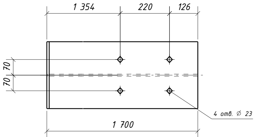
Дет. 305
