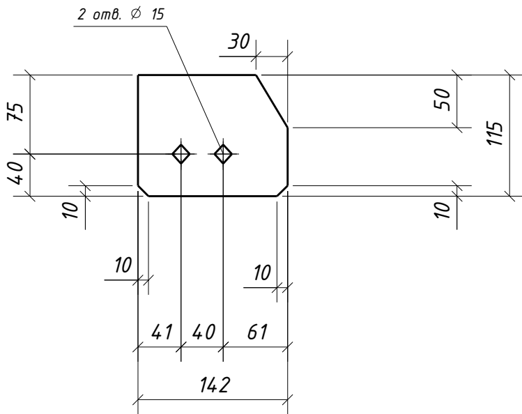
Дет. 428
