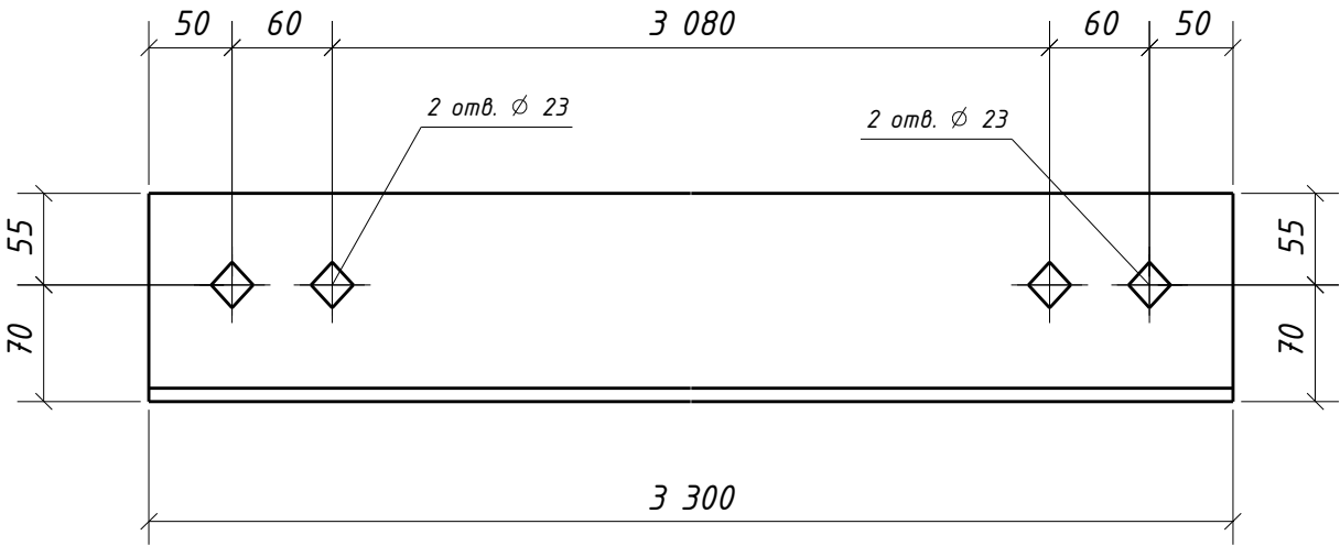
Дет. 558
