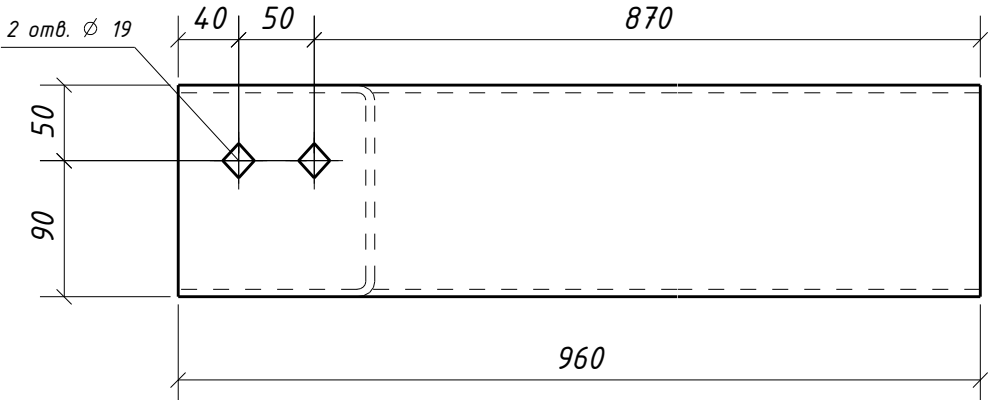
Дет. 650
