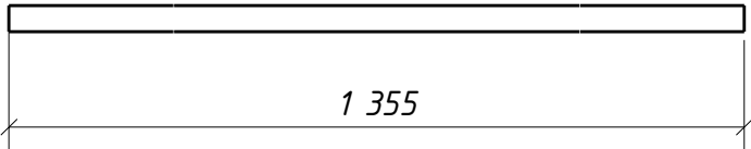
Развертка дет. 664
