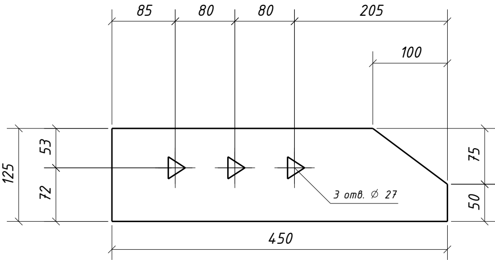
Дет. 68
