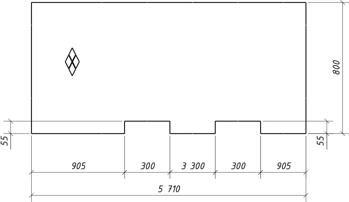
Дет. 790
