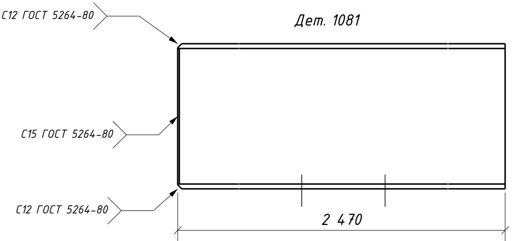
Вид снизу
