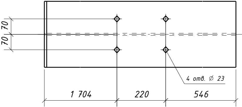
Вид снизу
